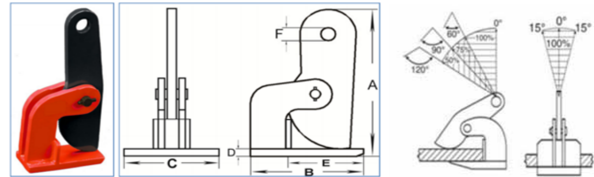
Achtung: Tragfähigkeit bei Schrägstellung- siehe Traglastdiagramm
