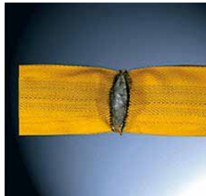
Rundschlinge-Proflix: nach 400 Scheuerintervallen
