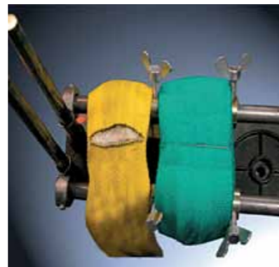
Vergleich Rundschlinge-Proflix und -Duplix Innox: nach 300 Scheuerintervallen
