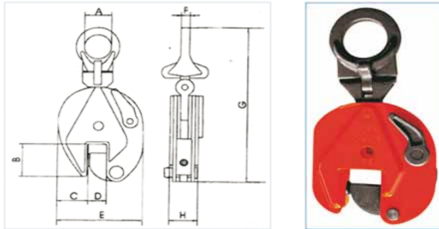
Blechgreifer mit 45° Schwenkbügel Tragfähigkeit: 500 – 5.000 kg
