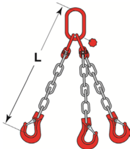
Anschlagketten GK10 3-Strg. nach DIN EN 818-2 konfektioniert mit Sicherheitslasthaken
