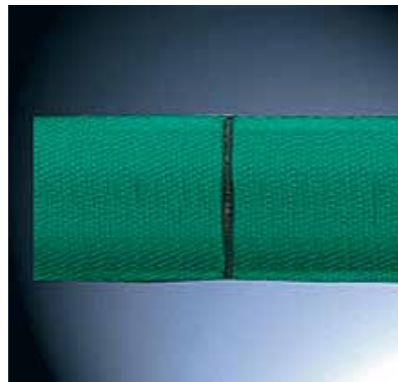
Rundschlinge-Duplix Innox: nach 400 Scheuerintervallen
