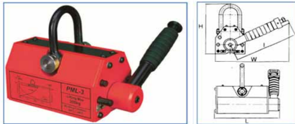
Permanent Lasthebemagnet Tragfähigkeit: 100 – 3.000 kg
