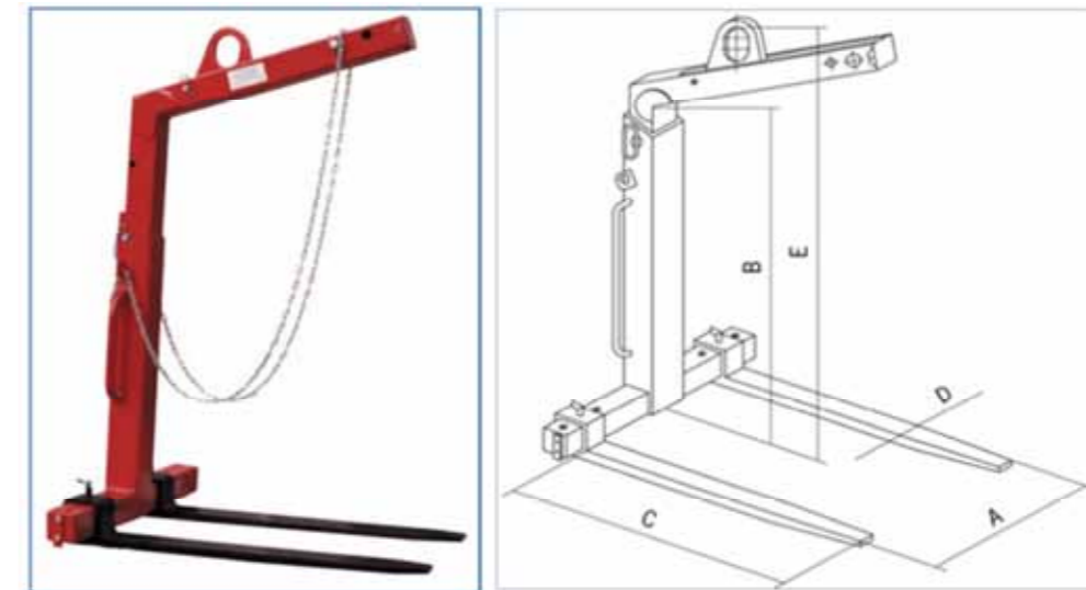
Ladegabeln Tragfähigkeit: 1.500 – 3.000 kg
