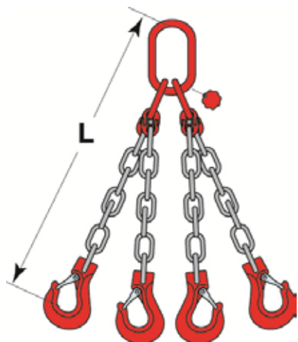
Anschlagketten GK10 4-Strg. nach DIN EN 818-2 konfektioniert mit Sicherheitslasthaken
